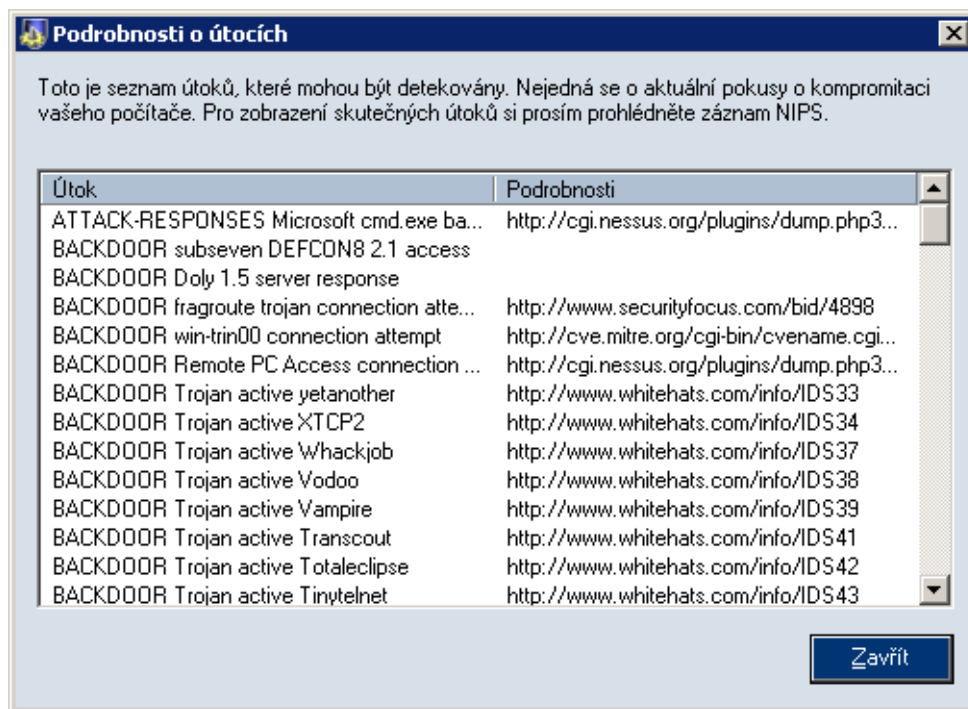
Obrázek 11.2 Detekce útoků — podrobnosti o útocích, které Kerio Personal Firewall dokáže zachytit
