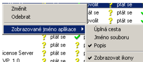
Obrázek 7.4 Pravidla pro aplikace — kontextové menu
