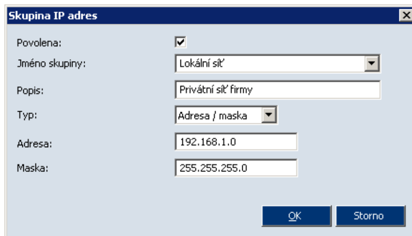
Obrázek 8.18 Paketový filtr — přidání položky do skupiny IP adres nebo vytvoření nové skupiny
