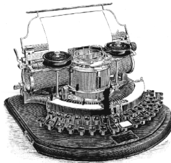
5. Psací stroj Hammond.
