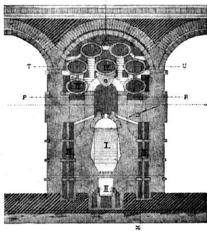
Příčný řez EFGH.
