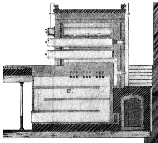
Podélný řez KLMNO.
