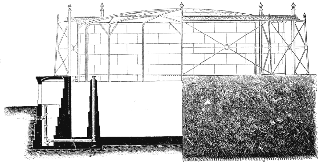
Plynojem se zděnou nádržkou (řez a pohled).
