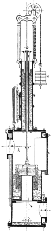
Kondensátor system »Pelouze a Audouin«.
