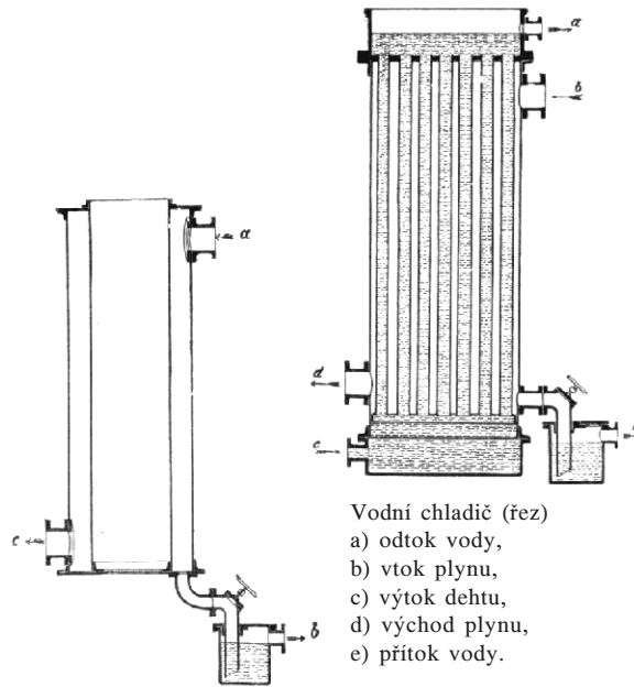
Vzdušní chladič (řez) a) vchod plynů, b) odtok dehtu, vody čpavkové, c) východ plynu.
