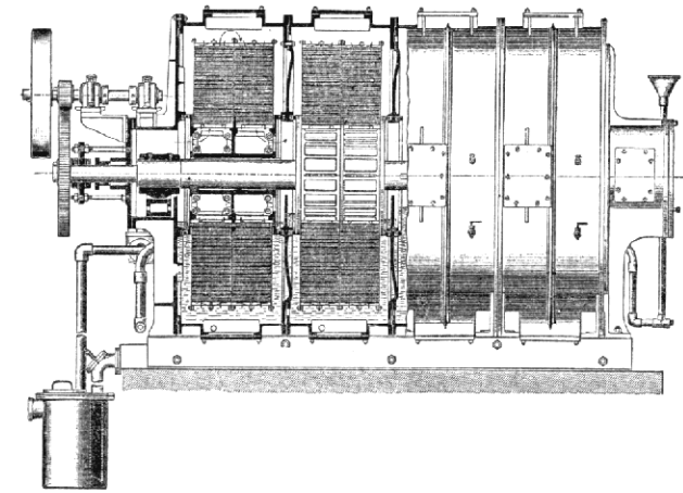
Standard skrubber (řez a pohled).
