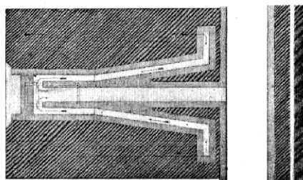
Řez kouřovými kanály.
