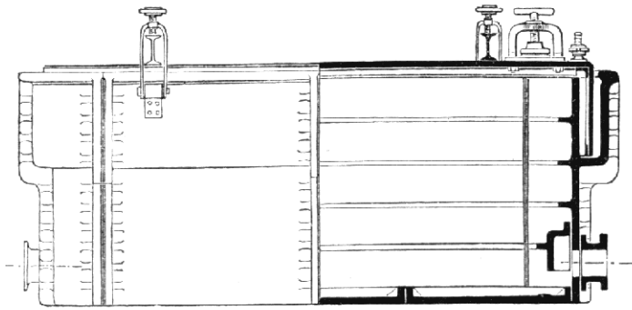
Čistič plynu (řez a pohled).
