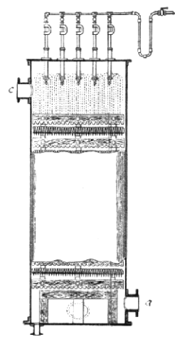
Skrubber s dřevěnými lískami (řez) a) vchod plynu, b) přítok vody, c) východ plynu.
