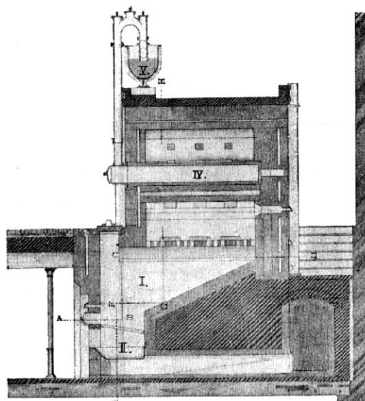
Podélný řez středem pece.
