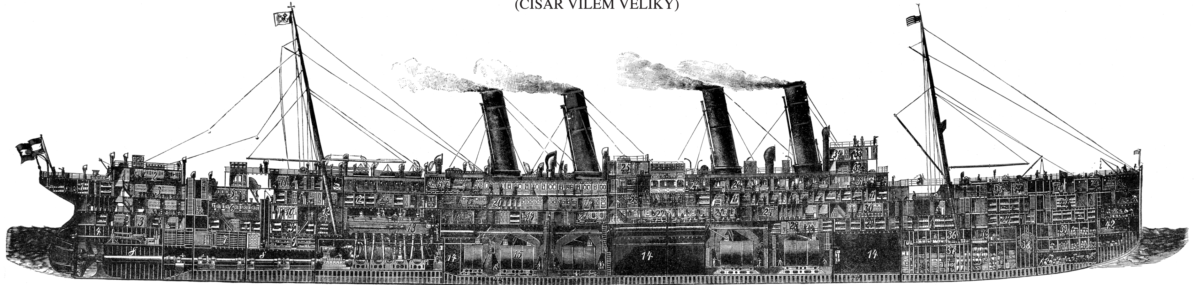
Řez podélný.
