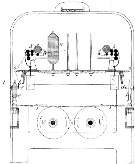
Č. 3326. Prstencový stroj přádací.
