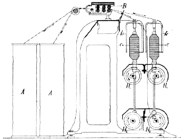
Č. 3325. Flyer na bavlnu.
