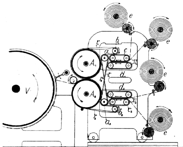
Č. 3329. Rozdělovadlo rouna (Josephyovo).
