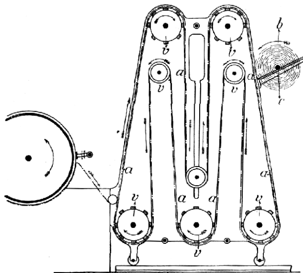
Č. 3328. Martinův listovací přístroj.
