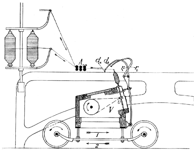
Č. 3327. Selfactor na bavlnu.
