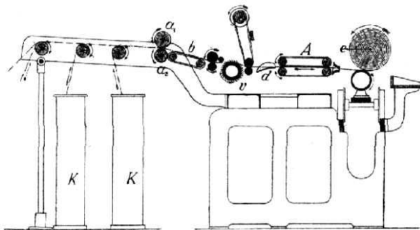
Č. 3332. Druhý posukovací stroj na vlnu česanou (stolice konvová).
