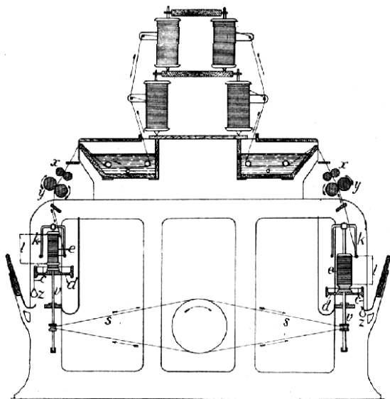
Č. 3334. Mokrý stroj přádací na len.
