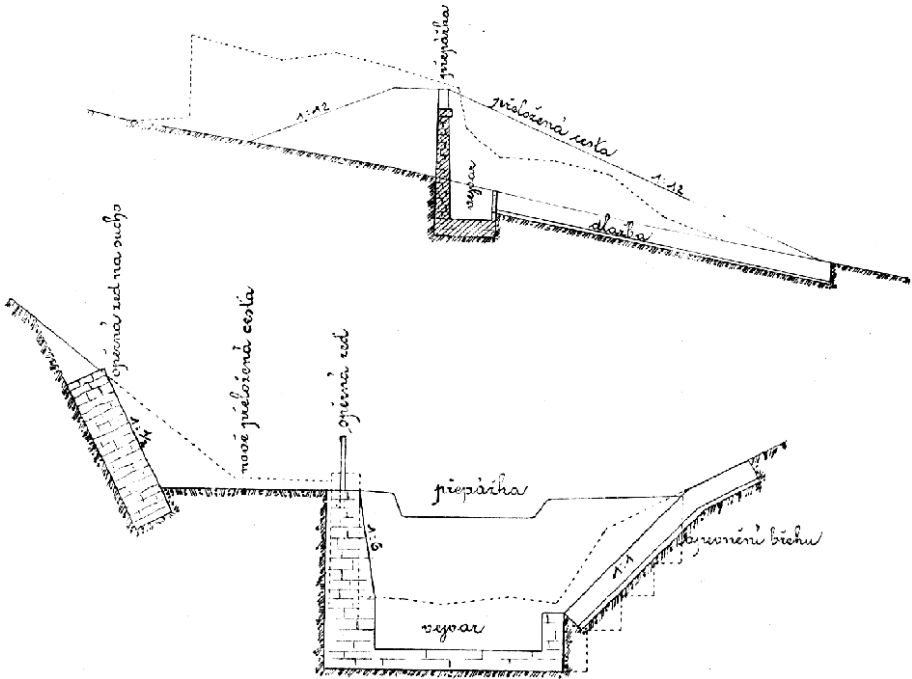
Č. 3336. Přehrada na potoku Lipenci.
