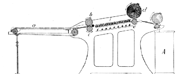
Č. 3333. Příkladací stroj na len.
