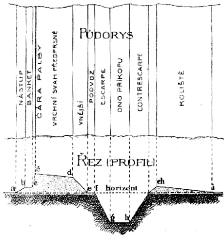
Č. 3335. Předprsen s příkopem. abcdě předprsen, ab nástup na banket, bc banket, cd vnitřní svah předprsené, cd vrchní svah předprsené (plongé), de vnější svah předprsené, ef podvoz (berma), fg hch příkop, fg escarpe, gh dno příkopu, hch contrascarpe, chi koliště.
