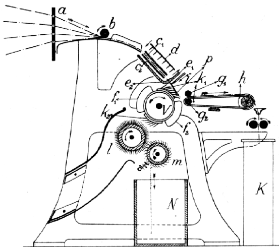
Č. 3331. Heilmannův stroj česací.
