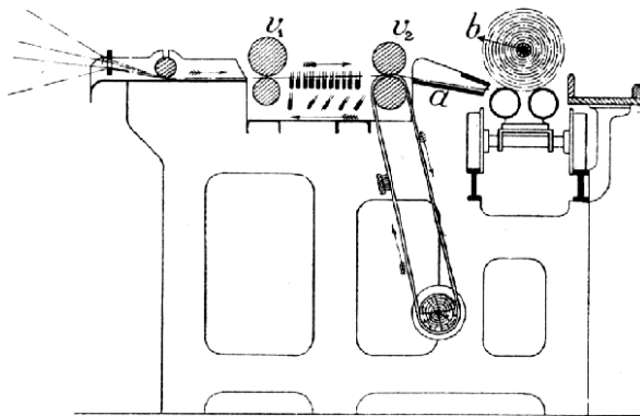
Č. 3330. První stroj posukovací na vlnu česanou.
