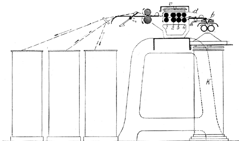
Č. 3324. Posukovací stroj na bavlnu.
