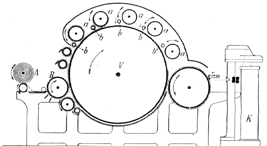
Č. 3323. Válcový stroj mykací.
