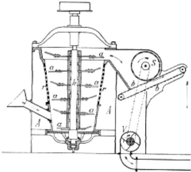
Č. 3315. Crightonovo čechradlo na bavlnu.
