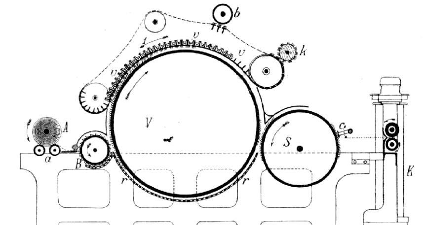
Č. 3322. Víčkový stroj mykací.
