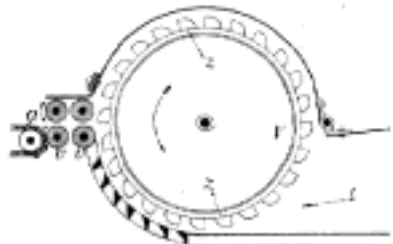
Č. 3316. Taylor Langovo čechradlo na bavlnu.
