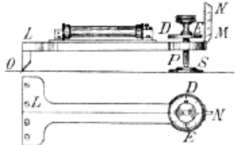
Č. 3308. Pravítko rektifikační.
