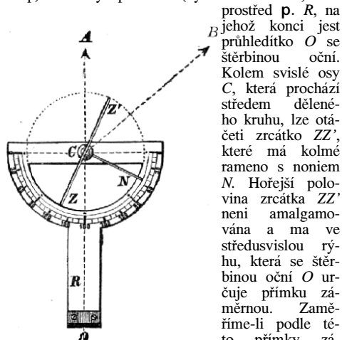
Č. 3303. Pravítko Falconerovo.
