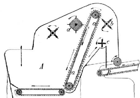
Č. 3318. Samočinný stroj nakládací.
