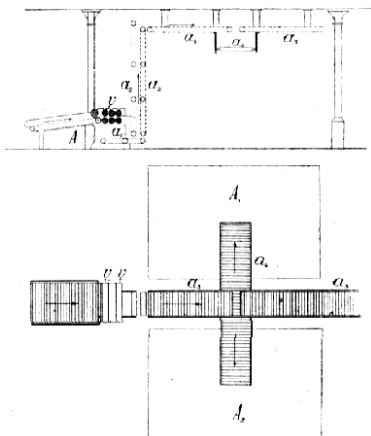
Č. 3314. Rozvolňovací stroj s mísmírou na bavlnu.
