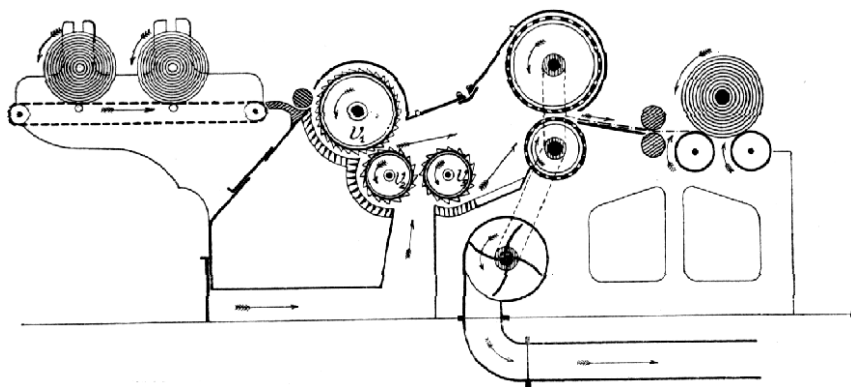
Č. 3319. Rislerův stroj.
