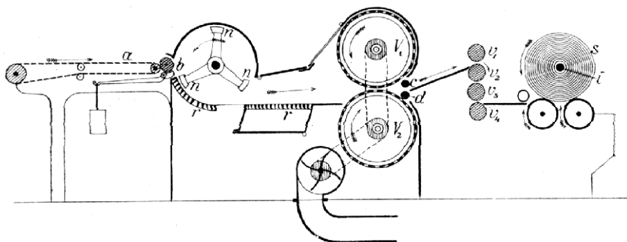
Č. 3317. Potěrací stroj na bavlnu.
