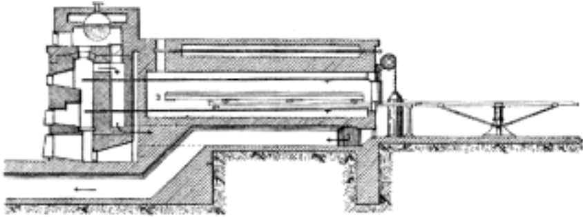
Č. 3076. Jednoduchá pec vytápěná horkou vodou.
