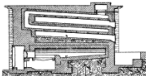
Č. 3075. Doberschinského pec se spodními tahy.
