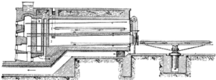
Č. 3077. Patrová pec vytápěná horkou vodou.
