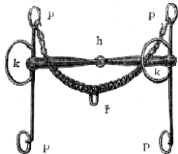
Č. 3078. Pelham. h hřídelek; pp, pp postraničky; f řetízek podbradní; kk kruhy postranní.
