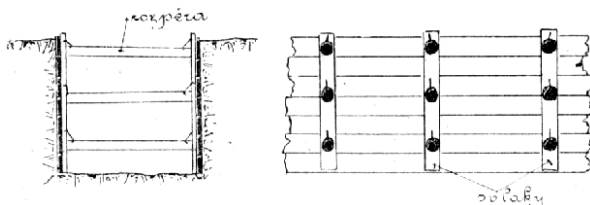
Č. 3064. Pažení obyčejné.
