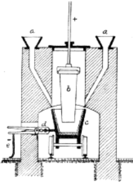
Č. 3071. Elektrická pec pro výrobu karbidu.
