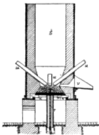
Č. 3069. Elektrická pec Urbanitzki-Fellnerova.
