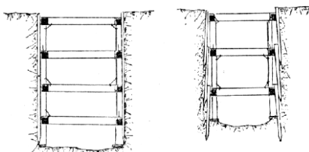
Č. 3065. Pažení hnané.
