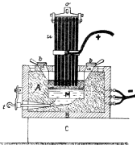
Č. 3068. Elektrická pec Héroultova.
