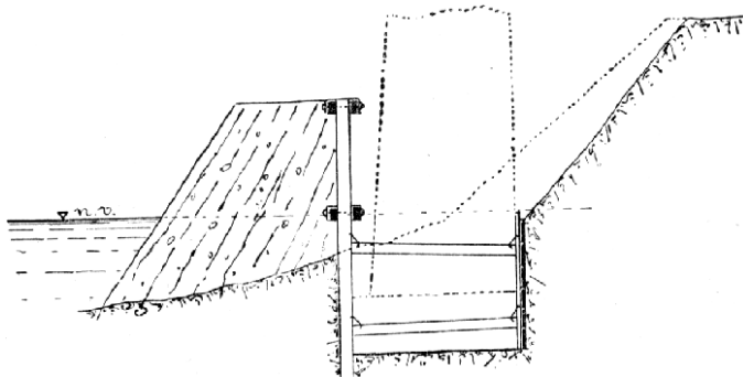
Č. 3066. Pažení pro pobřežní zed'.
