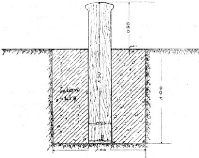
Č. 2989. Pachole dřevěné.
