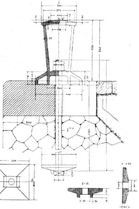
Č. 2990. Pachole železné.
