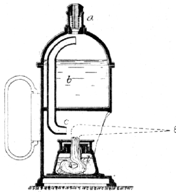
Č. 2993. Líhová lampa pájecí.
