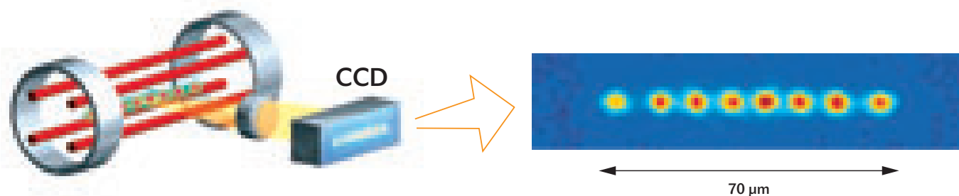
Obr. 1. V levé části obrázku je schéma lineární pasti používané na univerzitě v Innsbrucku. V ose pasti jsou drženy laserově vychlazené ionty. Vpravo je osmice iontů zviditelněná speciálním zobrazovacím zařízením. (Podle internetové prezentace R. Blatta, Universität Innsbruck, Institut für Experimentalphysik, http://online.itp.ucsb.edu/online/qinfo_co1/blatt/ )
