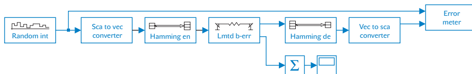
Obr. 1. Digitálny komunikačný systém s blokovým Hammingovým kódom
