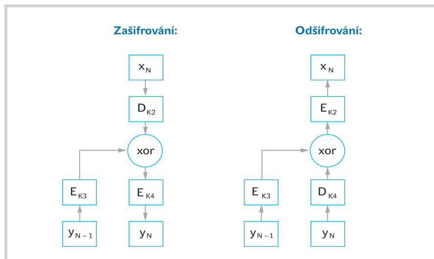
Obr. 3. Navrhovaná obrana
