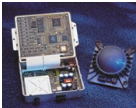
Počítač Bosch VP 44
