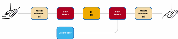
Obr. 4. Telefonování prostřednictvím IP sítě
