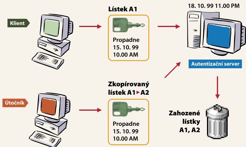
Obr. 2. Pomocí časových známek má server možnost ověřit platnost lístku a v případě expirace lístky zahodit.
