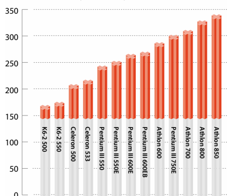
Celkový aplikační výkon – CHIP Mark
